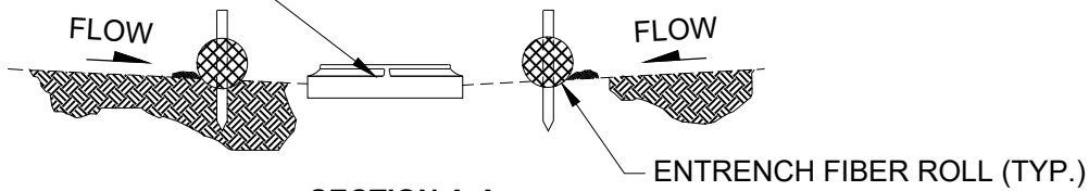
SECTION A-A
