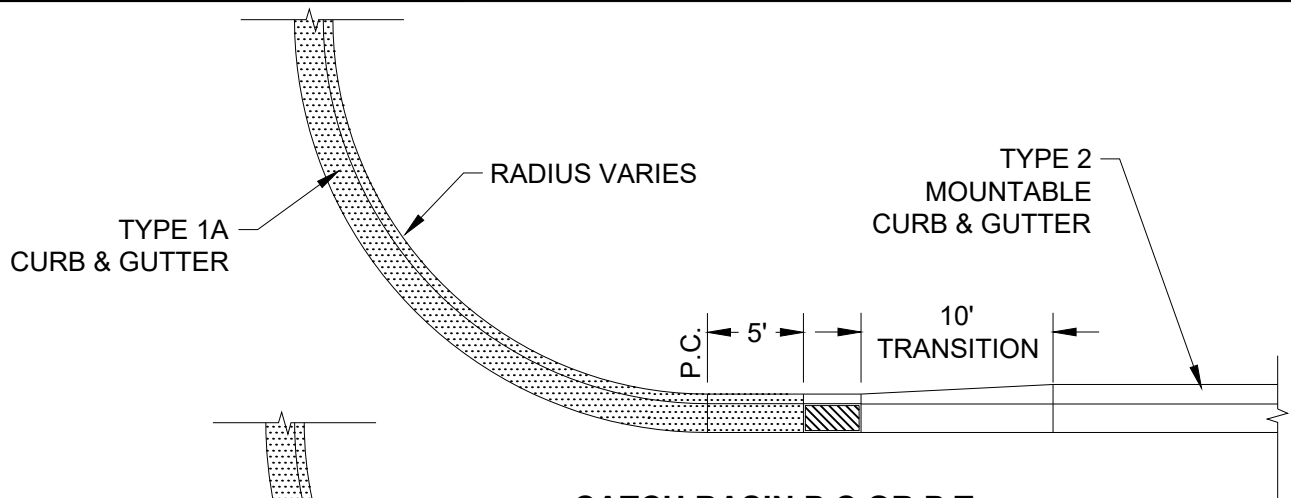
CATCH BASIN P.C. OR P.T.
