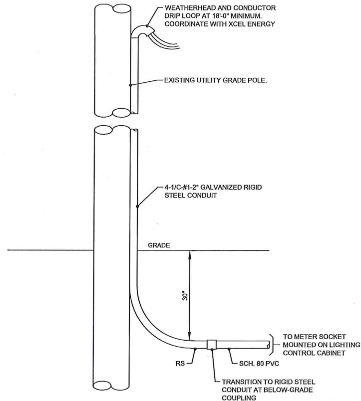
3 E2 SERVICE MAST DETAIL SCALE: N.T.S.
