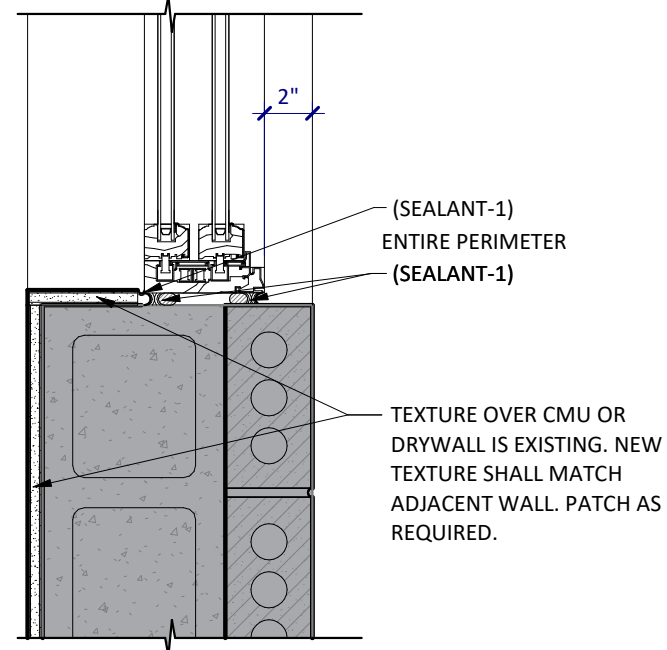
3B A311 WINDOW JAMB DETAIL SCALE: 1 1/2" = 1'-0"
